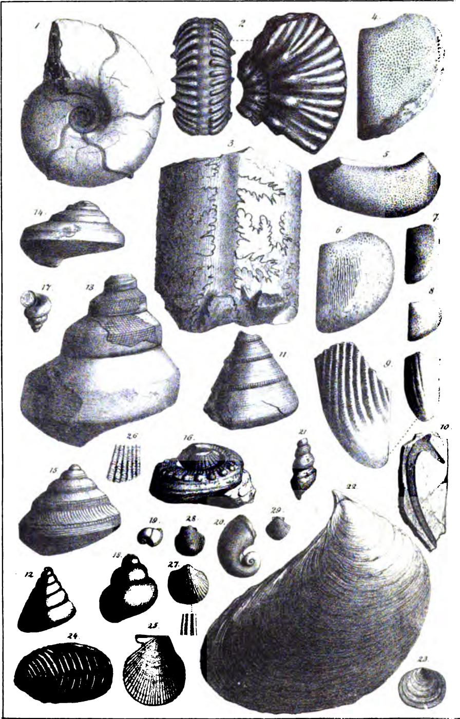
Quenstedt, Jura
